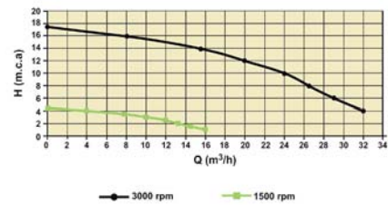
Curvas de rendimiento hidráulico Hydraulic performance curves Courbes de performances hydrauliques Curve delle prestazioni idrauliche
